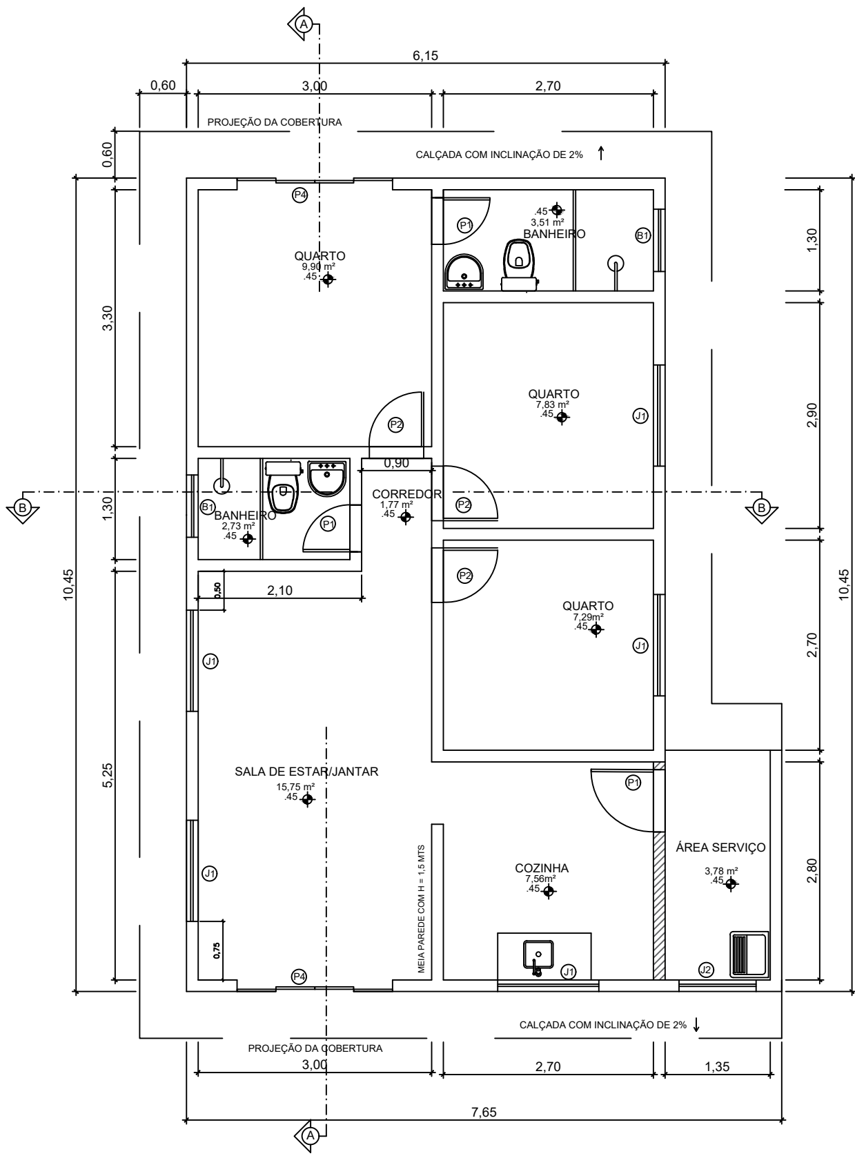
PLANTA BAIXA ESCALA: 1/50 ÁREA DE CONSTRUÇÃO: 68,92 m 2
